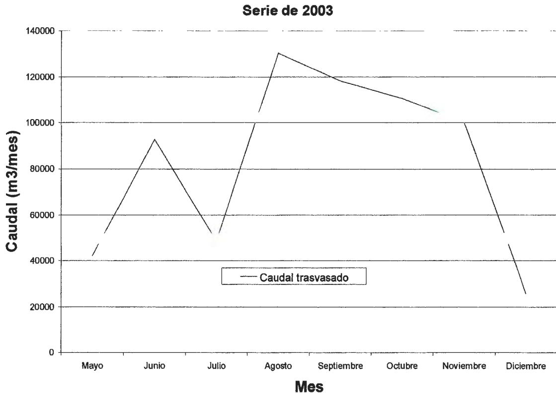
Figura 2.12. Caudal extraído de la quebrada Cortaderal
