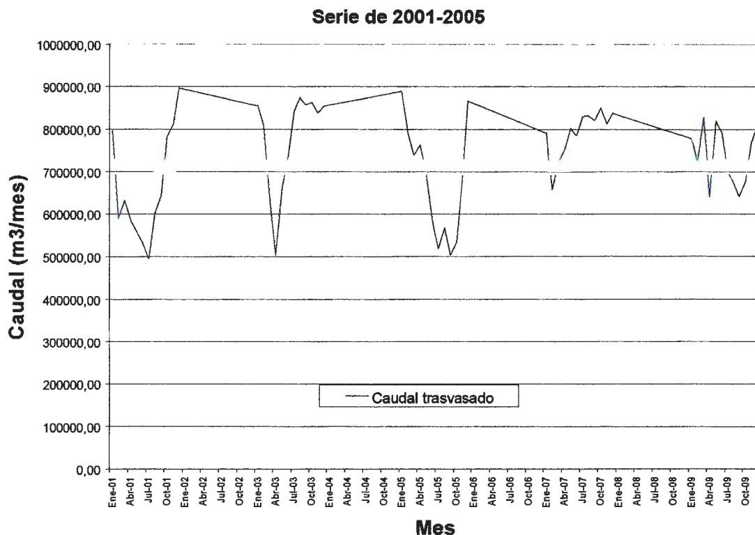
Figura 2.11. Caudal trasvasado de Teatinos
