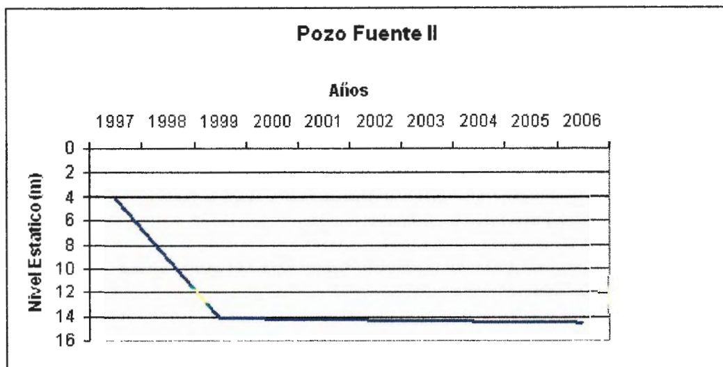
Figura 3.3. Comportamiento de los niveles de los pozos
