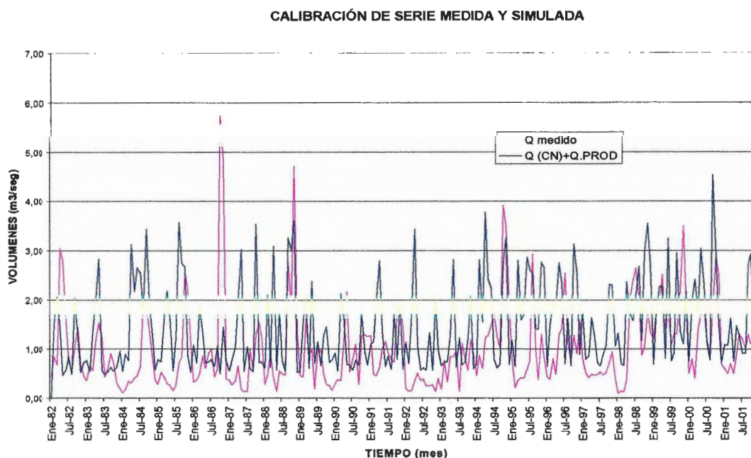
Figura 2.14. Caudal medido y caudal simulado
