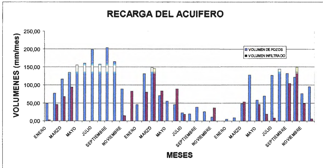
Figura 2. 17. Volúmenes de agua de pozos y de recarga
