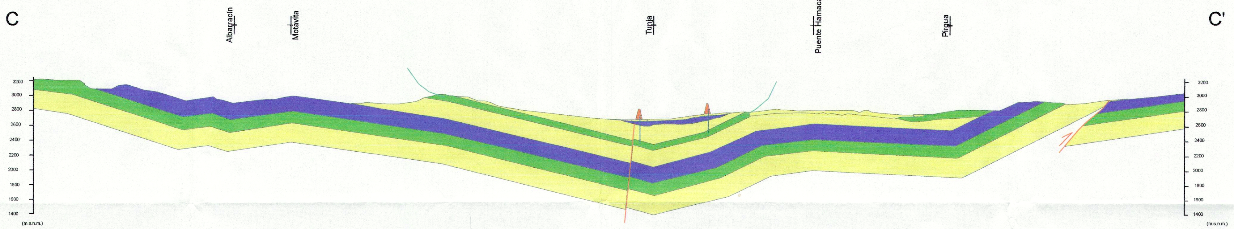
CORTE C - C'
