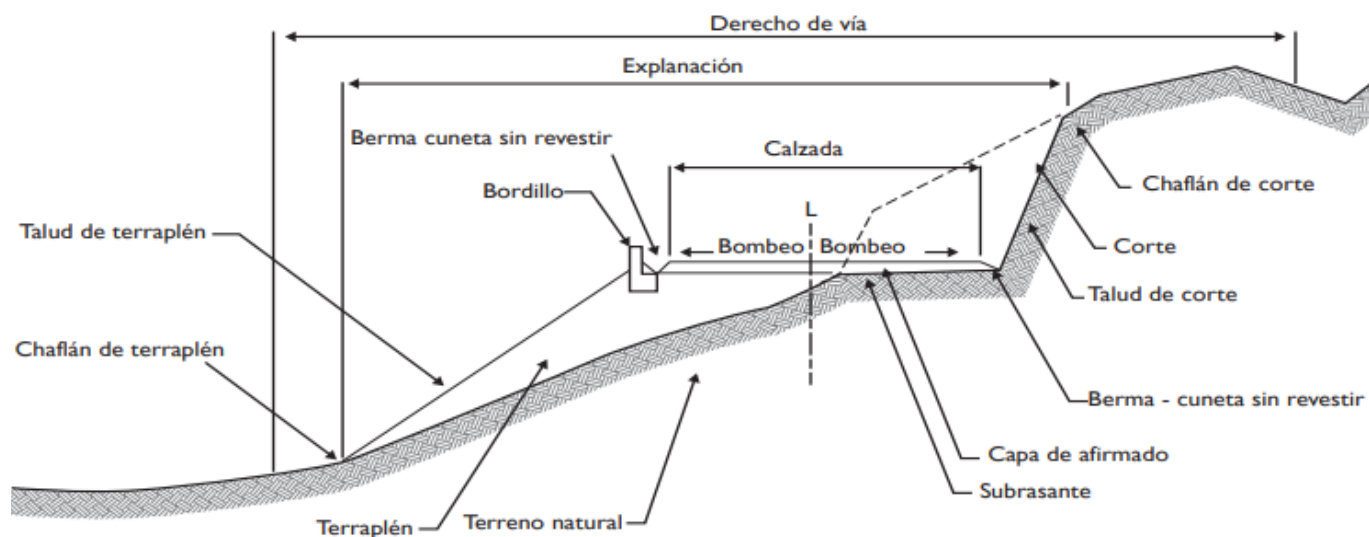
Figura 2. Sección transversal típica de la vía [20].
