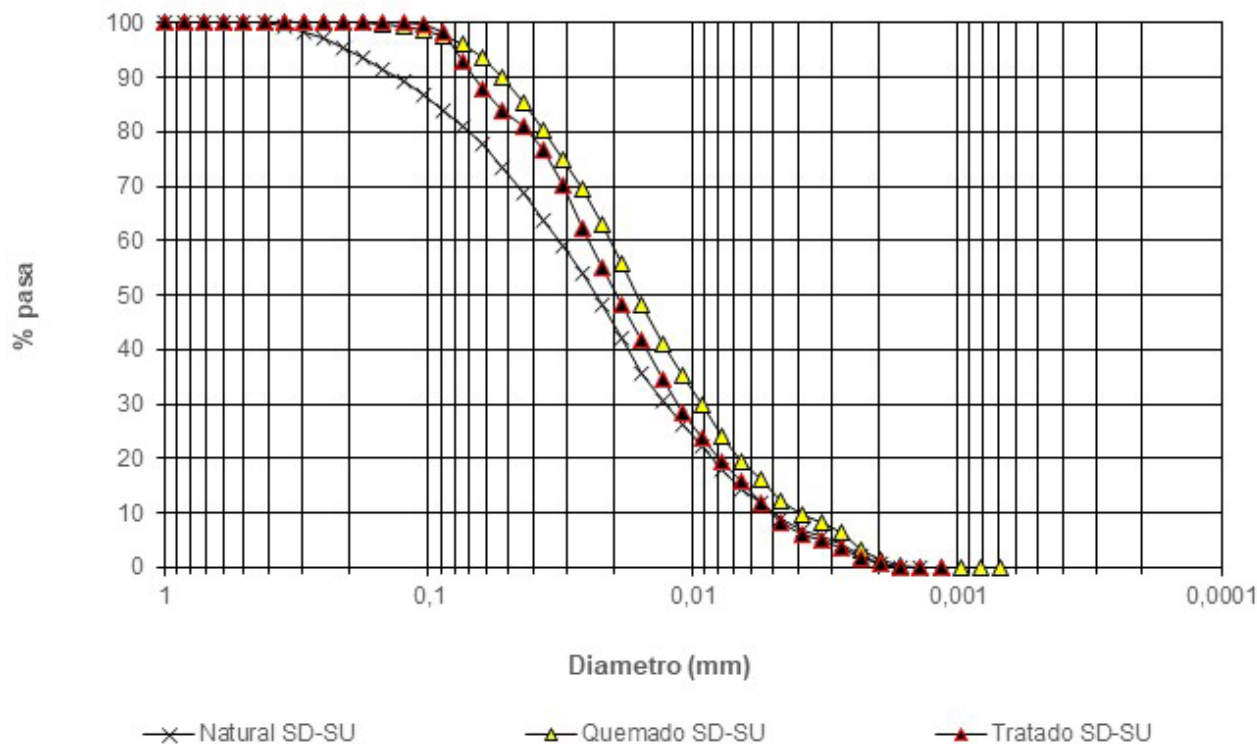
Figura 3. Curvas granulométricas del suelo natural, quemado y quemado-tratado sin uso de ultrason (SU) y sin defloculante (SD).
