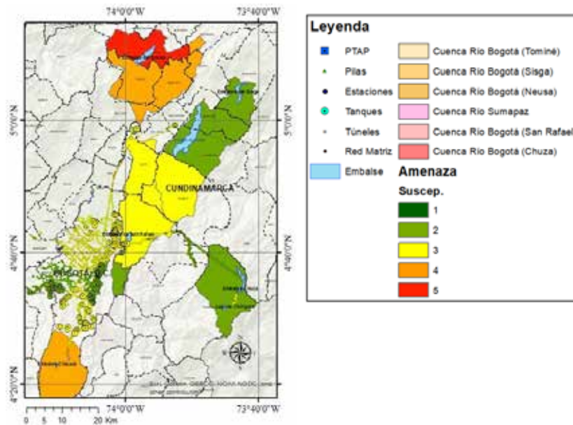
j) Vendaval
