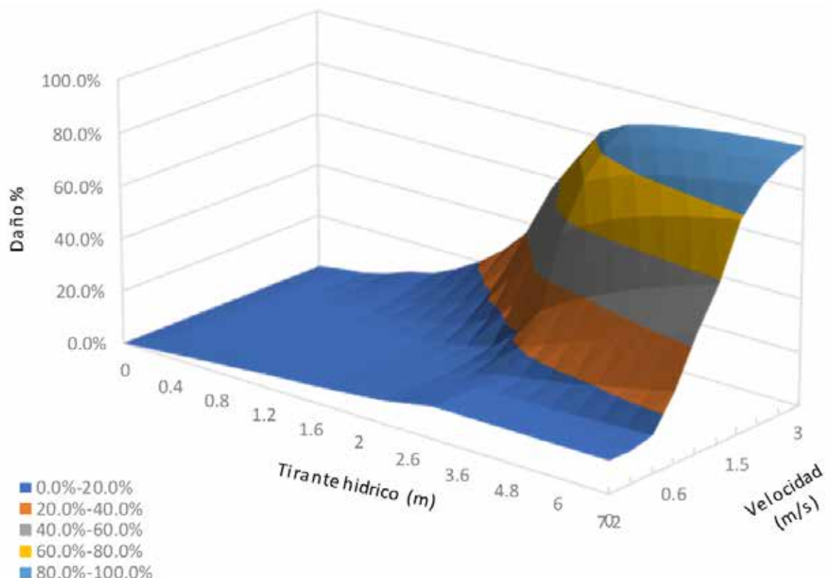
Figura 6. Ejemplo de función de vulnerabilidad para el rubro de edificaciones. Fuente: [8].
