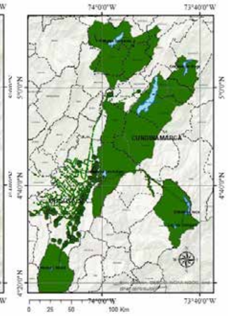
i) Volcanes
