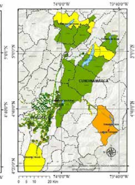
f) Deslizamiento
