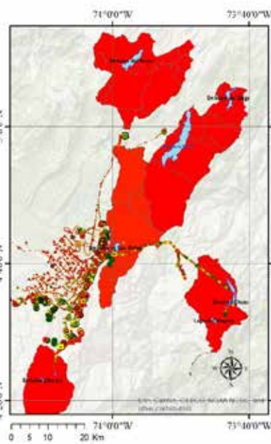
e) Inundaciones
