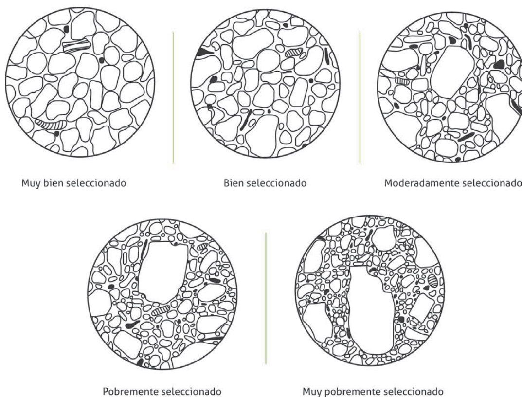
» Figura 10. Tabla de comparación visual para la clasificación de la selección (sorteamiento) de las partículas
