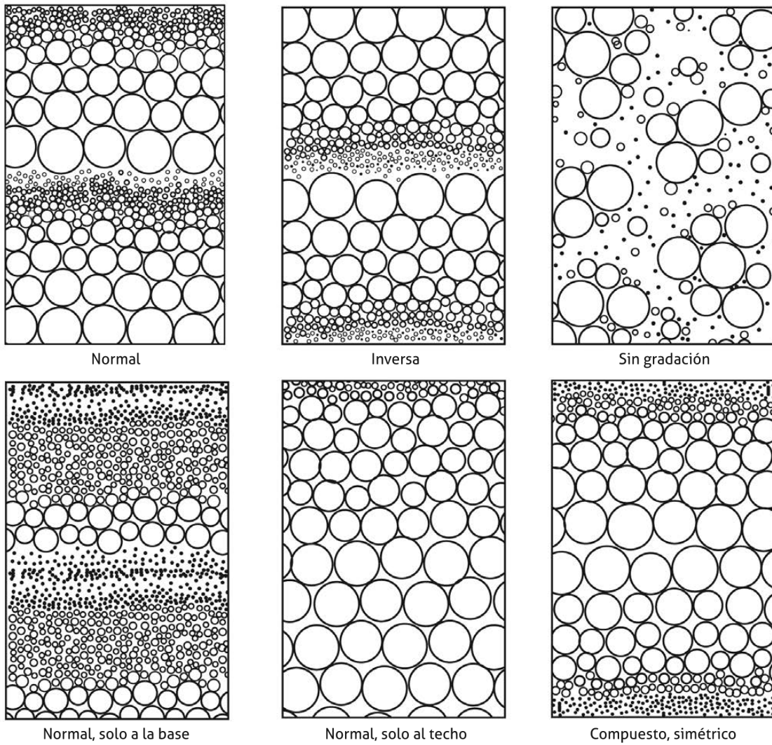
» Figura 8. Tipos de gradación
