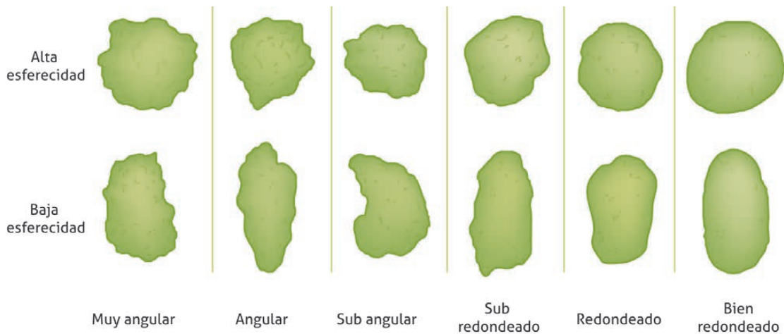
» Figura 6. Carta de comparación visual de la redondez y esfericidad de los clastos o granos
