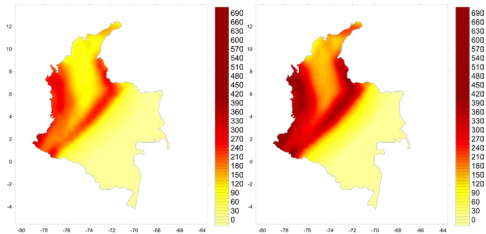
Figura 4. Mapas de amenaza uniforme para 475 años de periodo de retorno. Izq: aceleración máxima del terreno. Der: Aceleración espectral para 0.5 segundos. Aceleración en \text{cm/s}^2 .
