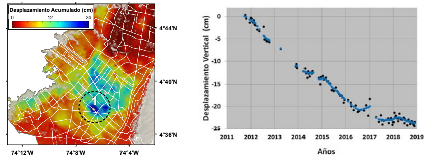
Figura 17. Mapa de desplazamientos acumulados del punto 1 sector Puente Aranda (izquierda). Serie de tiempo del Punto 1 (derecha).
