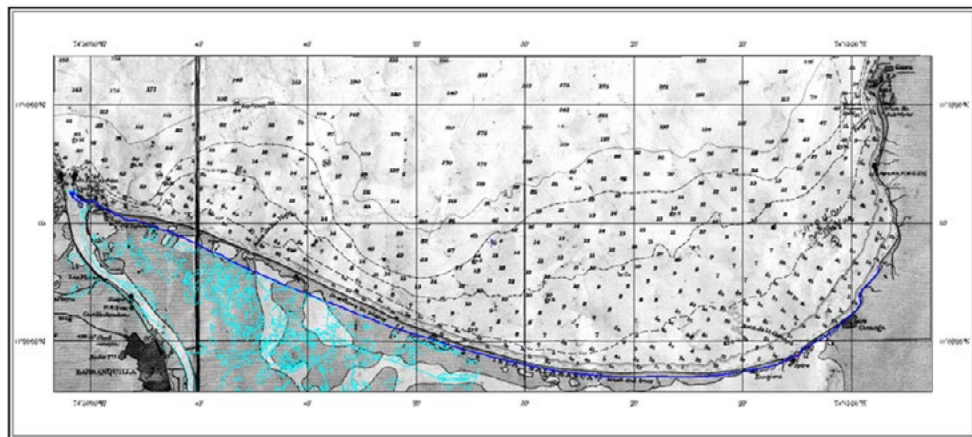
Figura 4. Retroceso costero (línea azul) con respecto a la cartografía del año 1944 en el sector de la Isla Salamanca. Se observa el efecto del déficit de sedimentos provocado por las obras de tajamares. Tramo: Barranquilla-Ciénaga. Fuente: [7].
