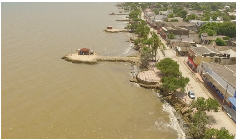
Figura 7. Fotos de obras de protección costera en el Golfo de Morrosquillo, donde se evidencia su obsolescencia. Arriba: Berrugas. Abajo: Santiago de Tolú. Fuente: propia.
