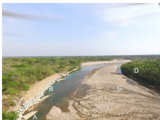
Figura 6. Vista panorámica del río Unete tomada con dron. Trabajo de campo efectuado en el río Unete en enero de 2018. (A) Espolones en concreto, (B) Estructura de contención con hexápodos, (C) Barra de sedimentos y (D) Terraza.
