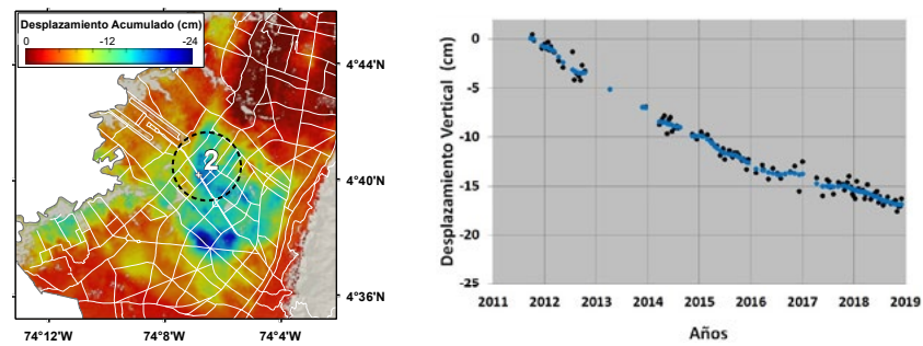
Figura 18. Mapa de desplazamientos acumulados del punto 2 (Normandía) (izquierda). Serie de tiempo del Punto 2, sector de Normandía (derecha).
