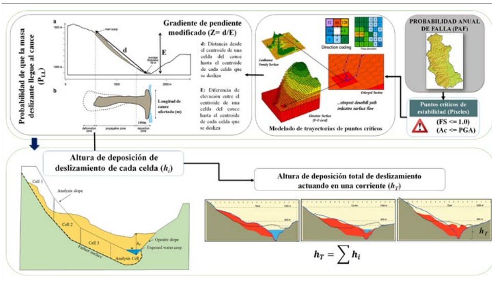
Figura 7. Esquema adoptado para el cálculo de la altura de depositación del movimiento en masa ( h_T ).
