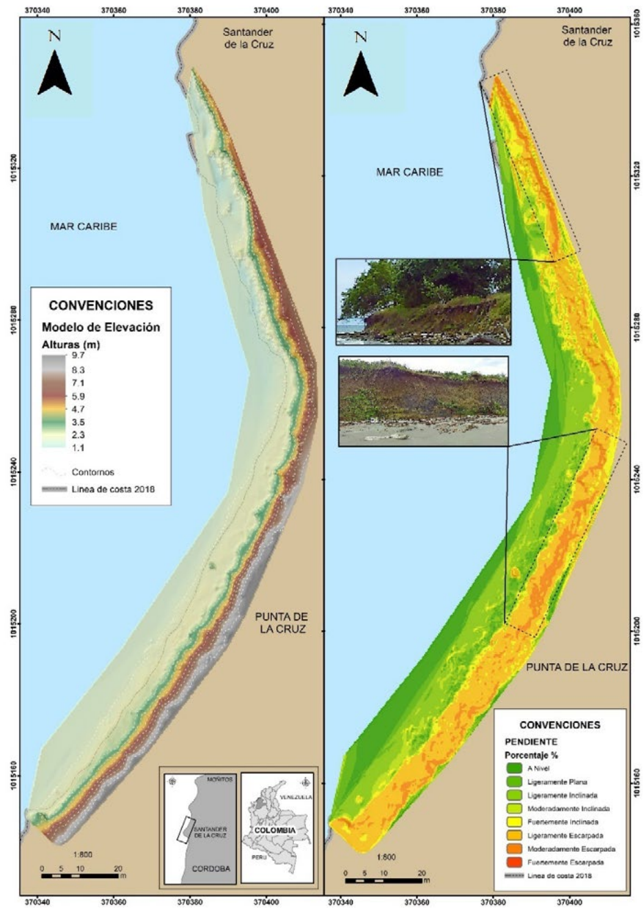
Figura 8. Modelo de elevación y pendiente en el sector acantilado de Punta de la Cruz.
