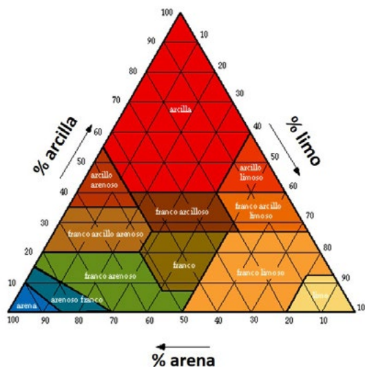
Figura 24. Triángulo de clases texturales básicas de suelos según el tamaño de partículas. Elaborado por el Departamento de Agricultura de los Estados Unidos (USDA).
