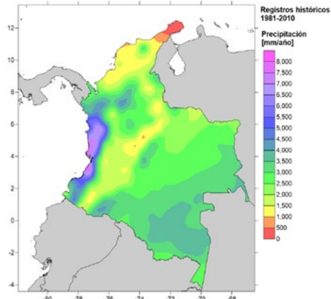
a) Precipitación Registros 1981 - 2010
