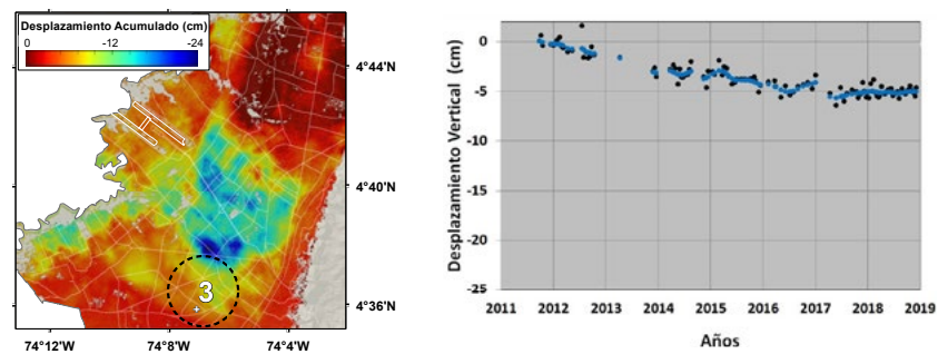
Figura 19. Mapa de desplazamientos acumulados del punto 3 (La Guaca) (izquierda). Serie de tiempo del punto 3 (derecha).
