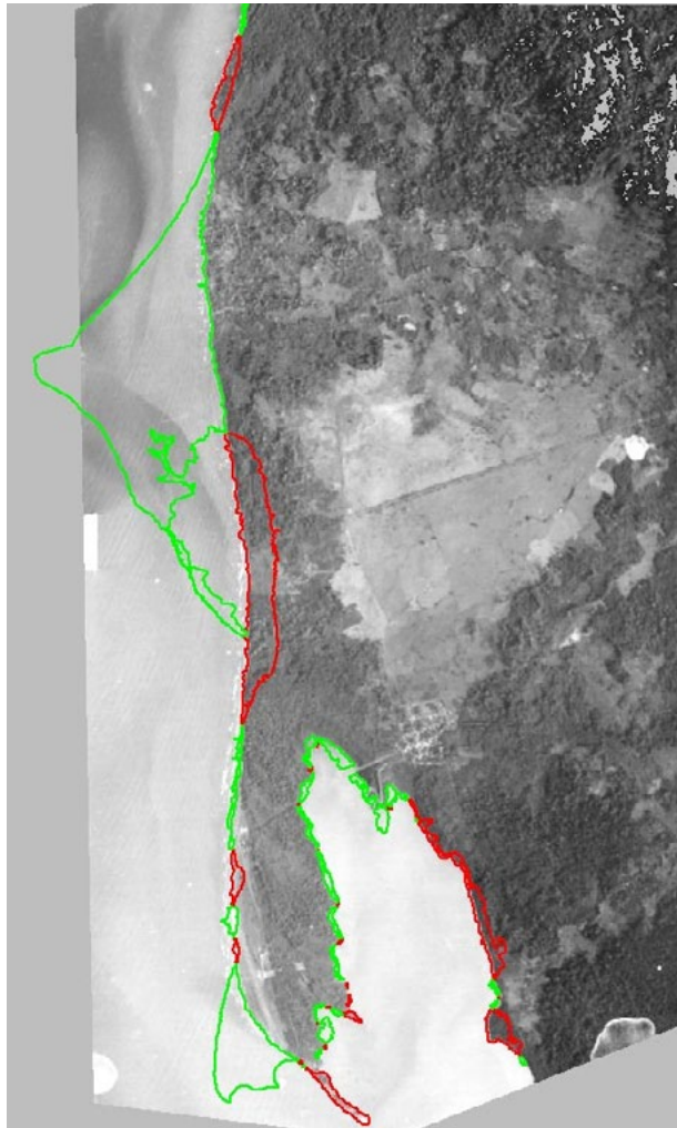
Figura 9. Variación de la línea de costa entre la desembocadura del río Turbo, la flecha de Yarumal y la flecha de Punta de Las Vacas entre 1946 (foto aérea) y 2005. (Golfo de Urabá). Los contornos en color representan áreas erosionadas (rojo) y sedimentadas (verde) [19].
