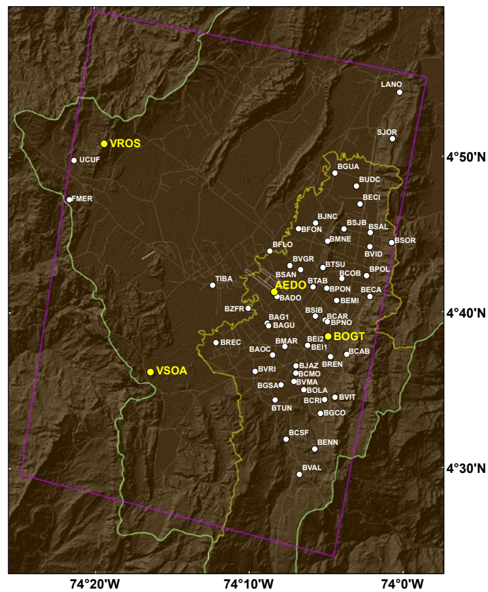
Figura 13. Mapa de localización de estaciones GPS empleadas para la integración con InSAR. Los círculos amarillos corresponden a estaciones permanentes, mientras los círculos blancos a estaciones de campo. El recuadro morado es la zona de cobertura de las imágenes TerraSAR-X empleadas.
