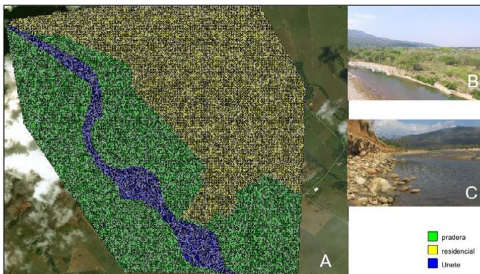
Figura 13. Usos de suelo en Iber. Los usos de suelo se determinaron a partir de las imágenes satelitales y las visitas realizadas a la zona del proyecto. (A) Usos de suelo identificados a partir de malla triangular no estructurada en el software Iber, (B) Terraza aluvial y (C) Material del lecho del río Unete.
