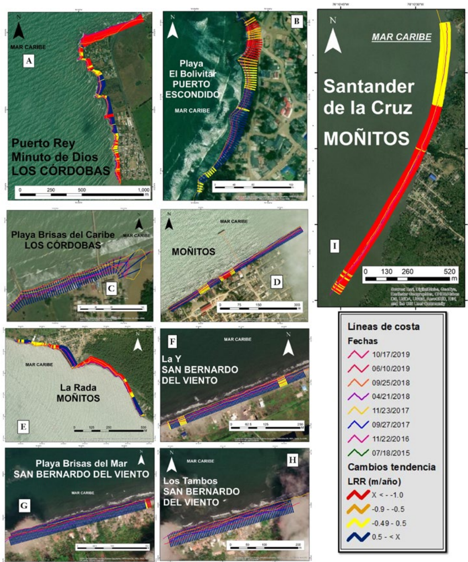
Figura 5 . Cambios en línea de costa tendenciales para las zonas de monitoreo del departamento. (A) Minuto de Dios y Puerto Rey, (B) playa El Bolívar, (C) playa Brisas del Caribe, (D) Moñitos, (E) La Rada, (F) La Y, (G) Brisas del Mar, (H) Los Tambos, (I) Santander de la Cruz. Clasificación: Muy Alta ( LRR < -1 m/año), Alta ( -1 > LRR > -0.5 ), Estable ( -0.5 < LRR > 0.5 ) y Acreción ( LRR > 0.5 ).
