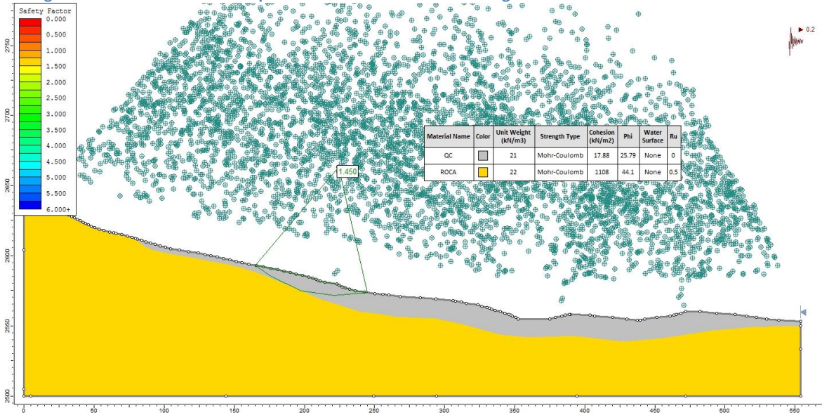
Figura 13. Distribución de los FS para el escenario con obras de mitigación en la condición extrema del Perfil E.
