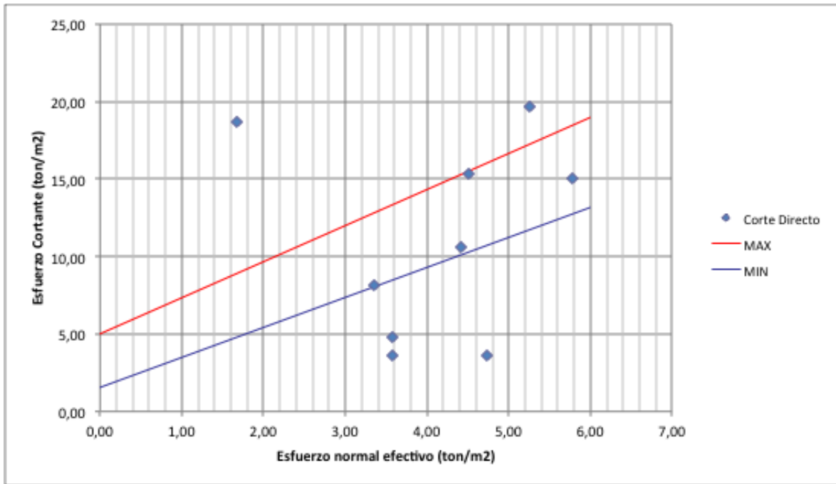
Figura 3. Análisis de los parámetros de resistencia (Sondeo 2)
