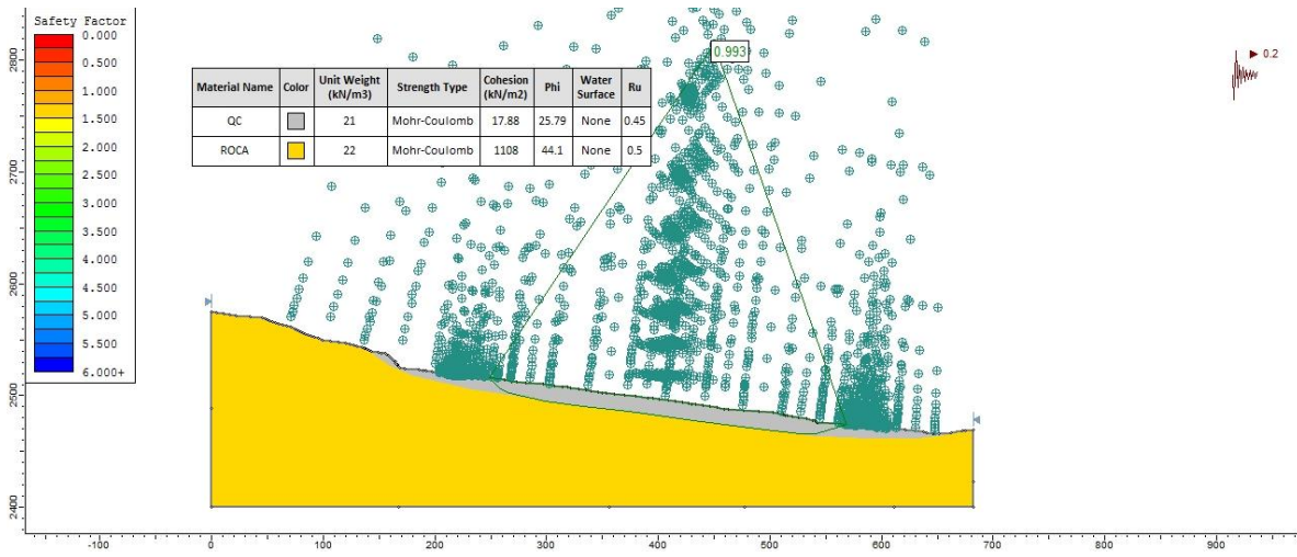
Figura 8. Distribución de los FS para el escenario actual en la condición extrema del Perfil E.
