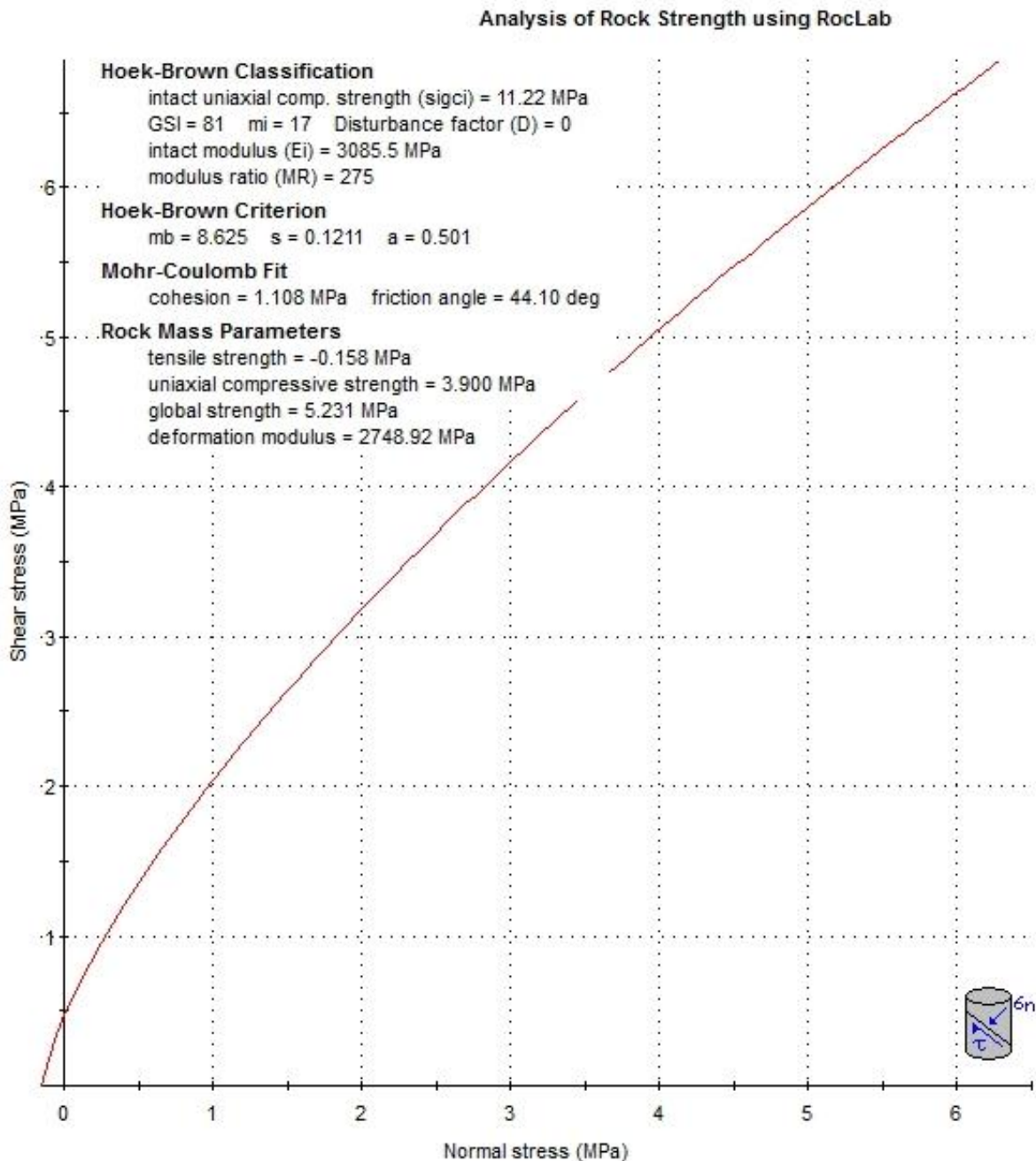
Figura 4. Salida gráfica del software RocLab 1.0 para la caracterización mecánica de la roca.
