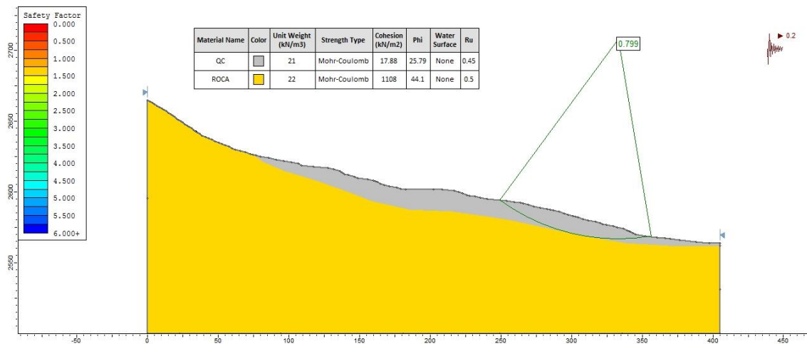
Figura 6. Distribución de los FS para el escenario actual en la condición extrema del Perfil C.
