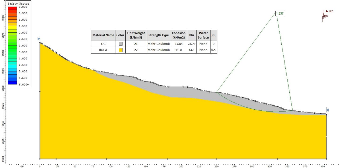
Figura 11. Distribución de los FS para el escenario con obras de mitigacion en la condición extrema del Perfil C.
