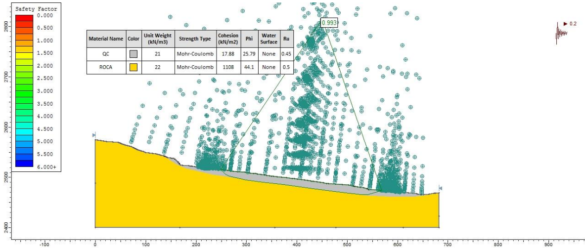
Figura 4. Distribución de los FS para el escenario actual en la condición extrema del Perfil E.
