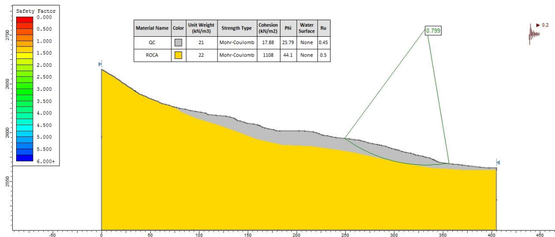
Figura 2. Distribución de los FS para el escenario actual en la condición extrema del Perfil C.
