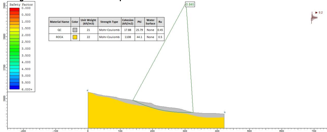
Figura 2. Distribución de los FS para el escenario actual en la condición extrema del Perfil C.
