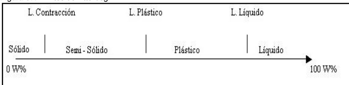
Figura 37. Límites de Atterbeg
