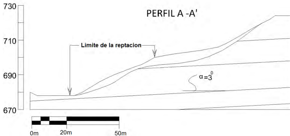
Figura 19. Esquema del movimiento, perfil desprendimiento 1
