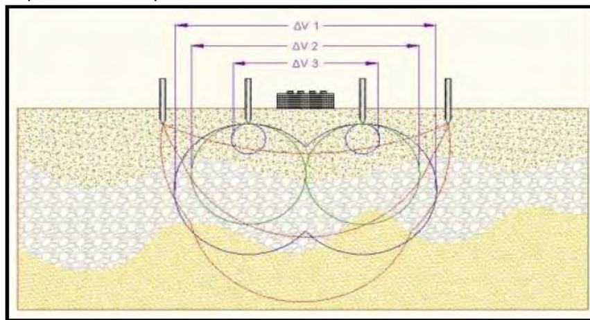
Figura 30. Principio teórico de operación de las TER's.
