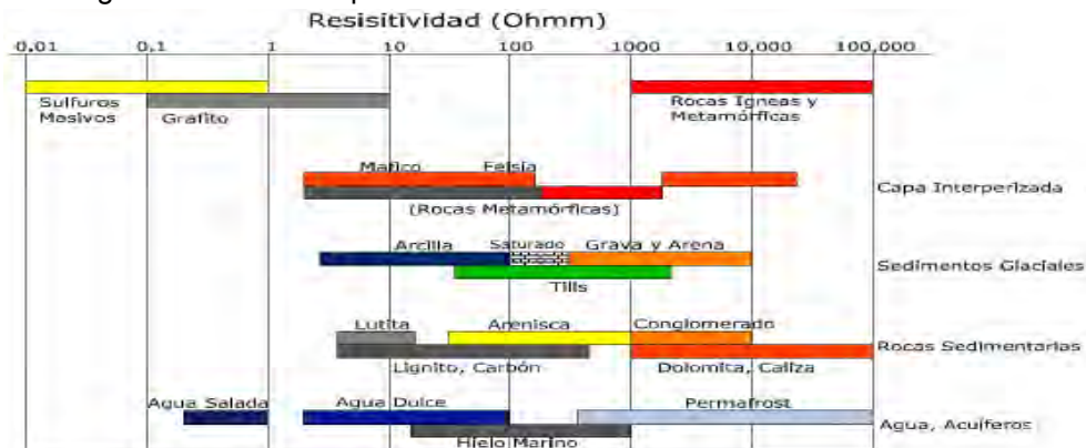
Figura 31. Rangos de resistividad para diferentes materiales.
