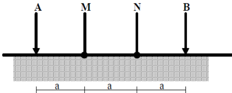
Figura 32. Dispositivo Wenner.
