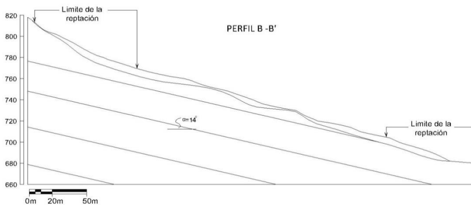
Figura 21. Esquema del movimiento, perfil desprendimiento 2
