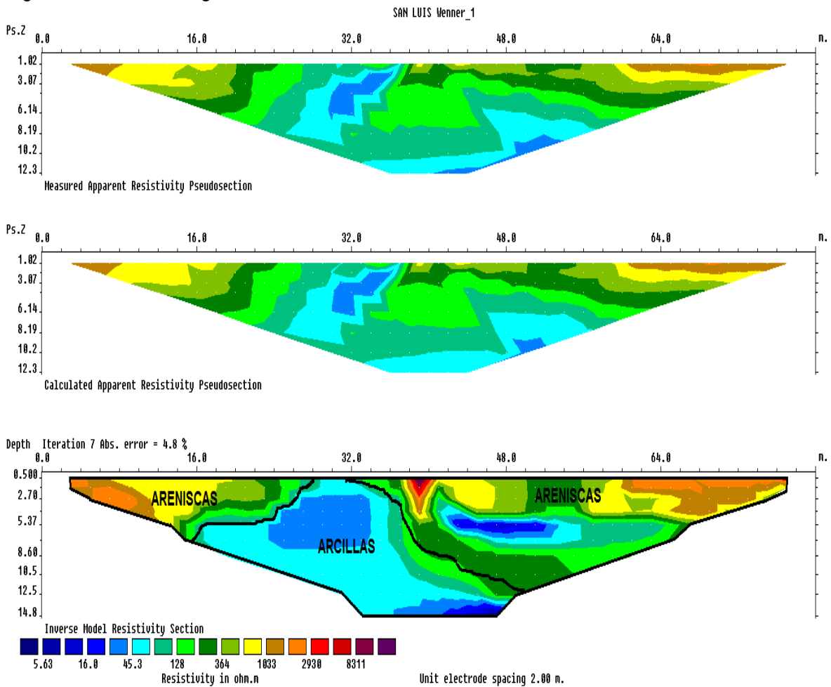
Figura 34. Perfil 1 tomografía.
