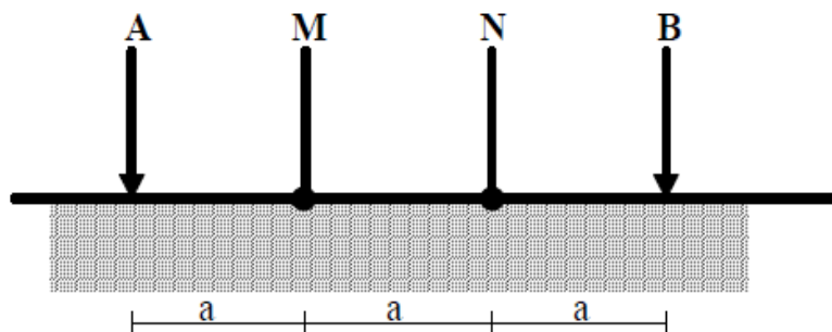
Figura 26. Dispositivo Wenner.
