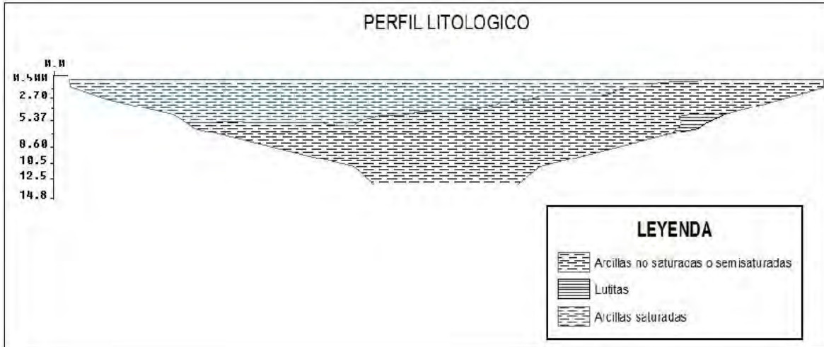
Figura 29. Perfil litológico 1
