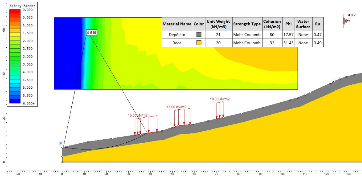
Figura 5. Distribución de los FS para el escenario actual en la condición extrema del Perfil 1.
