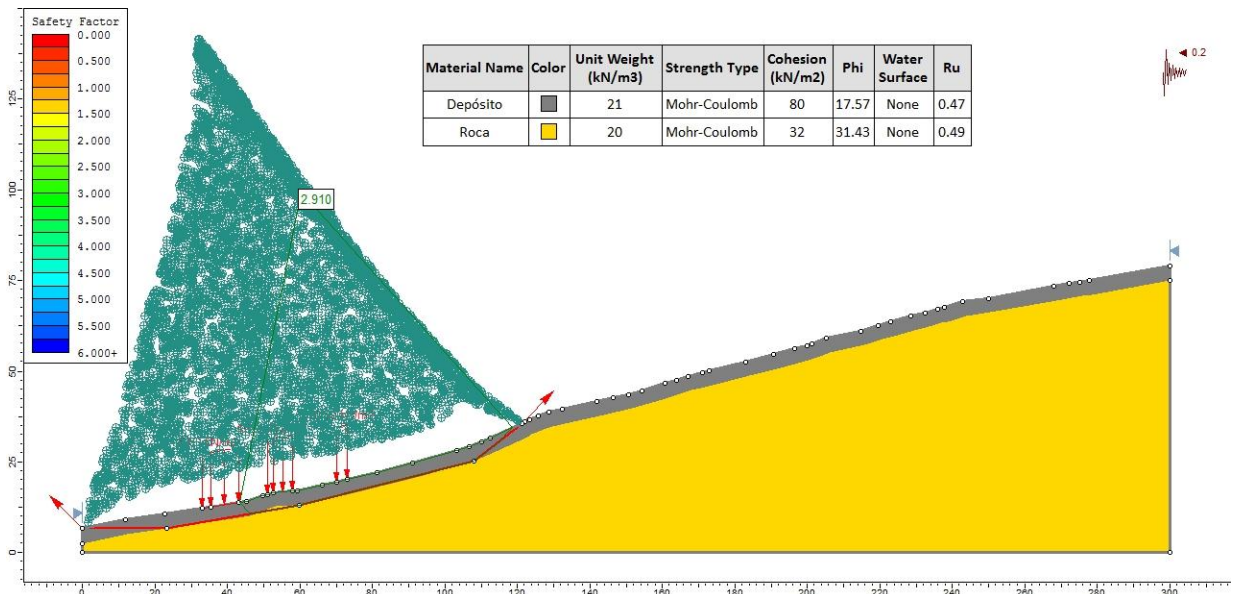
Figura 6. Análisis de falla planar para el escenario actual en la condición extrema del Perfil 1
