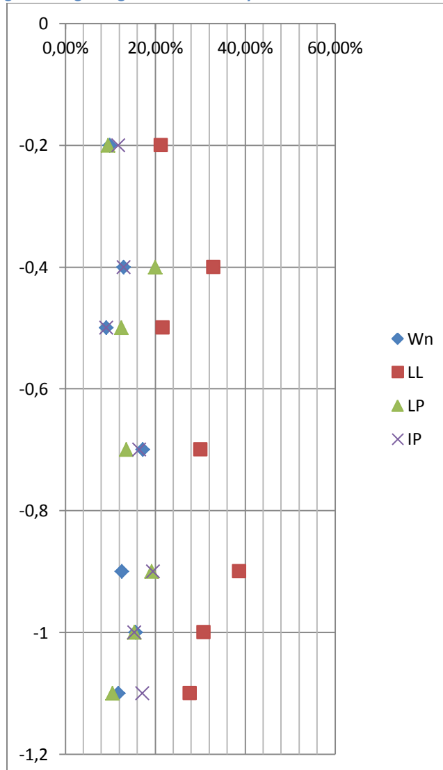
Figura 1. Registro gráfico de los ensayos de laboratorio del sondeo 2.
