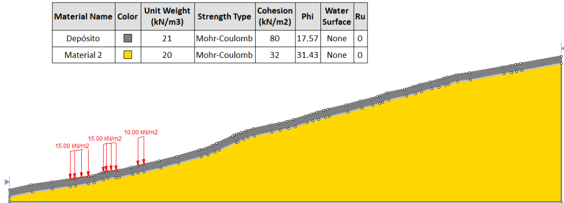
Figura 4. Modelo Geológico - Geotécnico Perfil 1.
