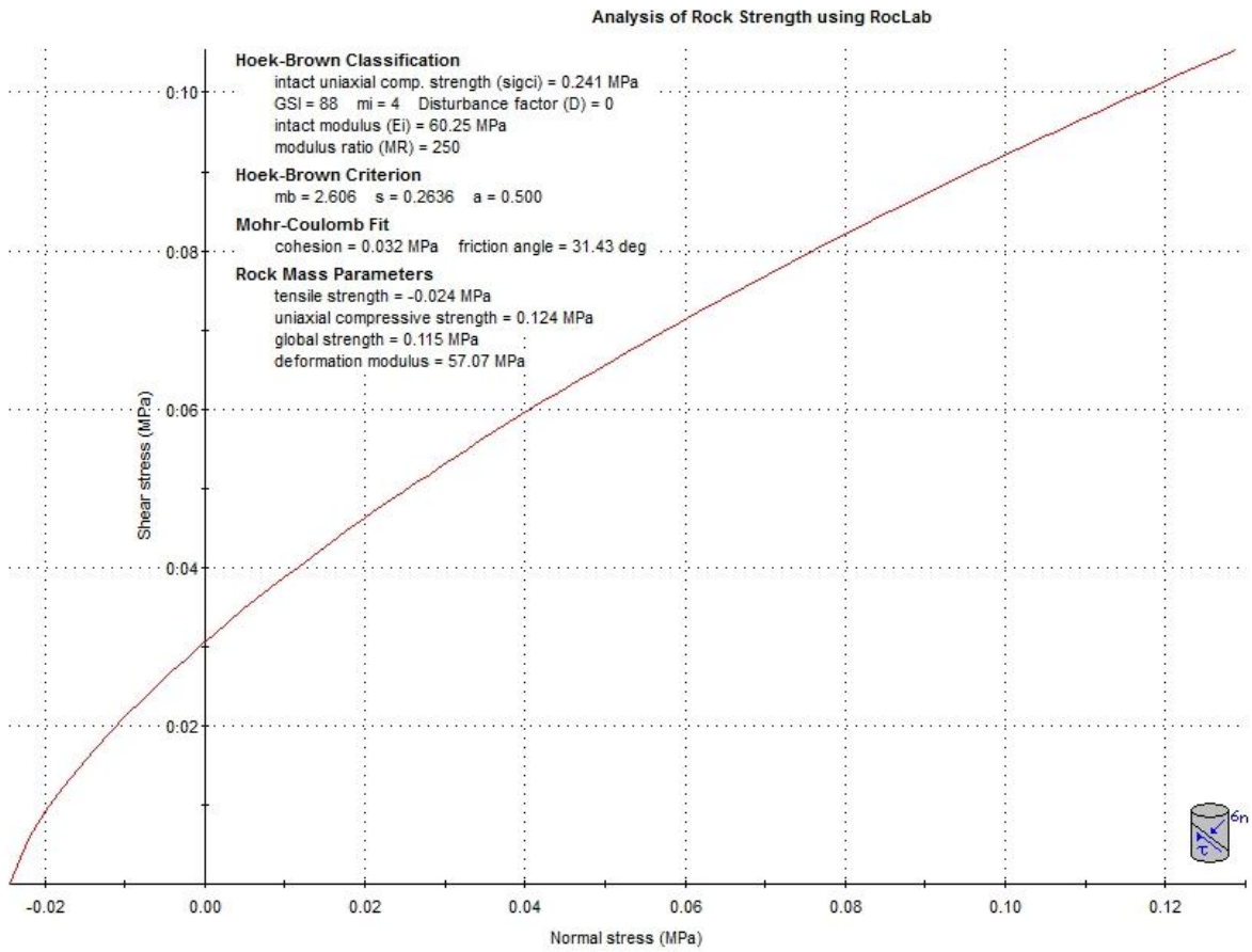
Figura 3. Salida gráfica del software RocLab 1.0 para la caracterización mecánica de la roca.
